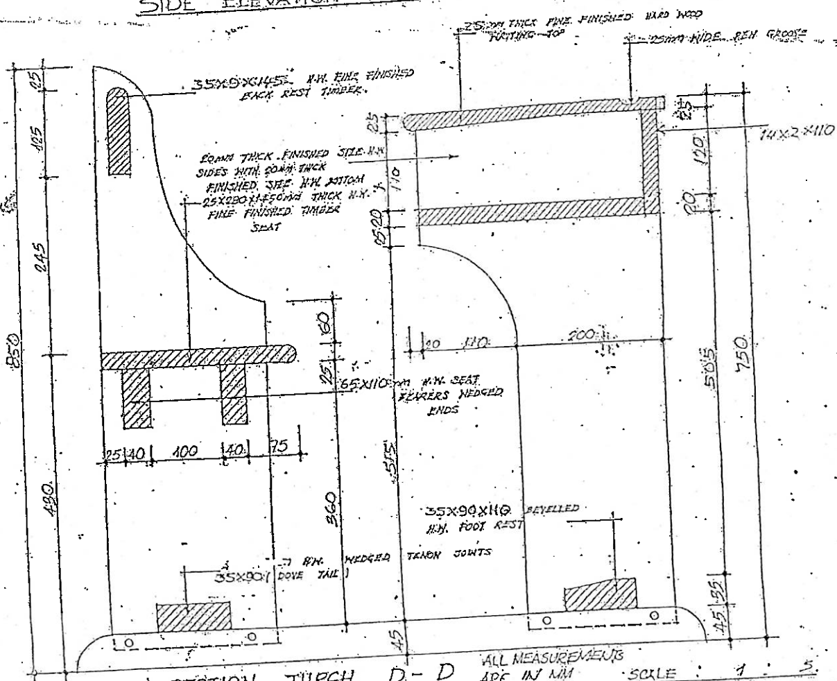
SIDE ELEVATION (MEDIUM)
